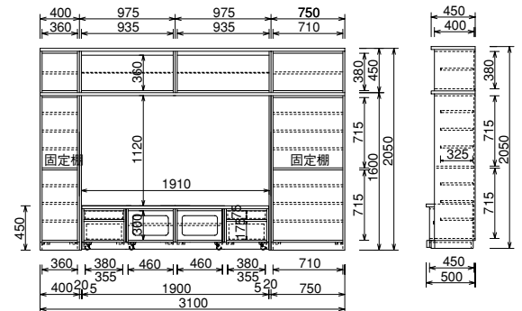
TVボードは配線がしやすいようにキャスター付きになっています。 ※安定性の為D40にはキャスターが付きません。
