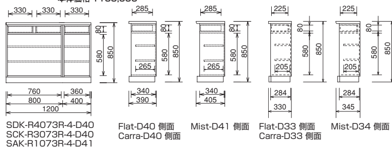
Flat カウンターボード SDK-R4073R-4-D40 CB サイズ : W1200・D390・H850 本体価格 ¥155,000
